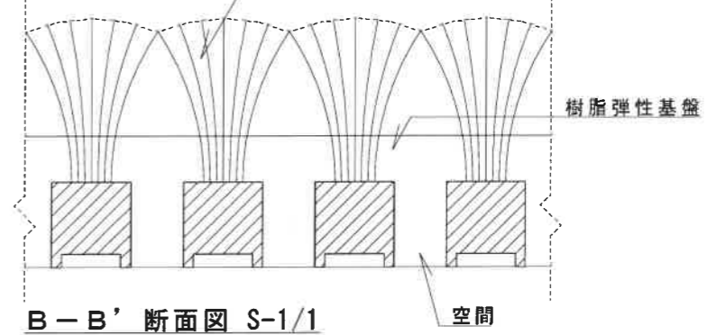
B-B' 断面図 S=1/1
