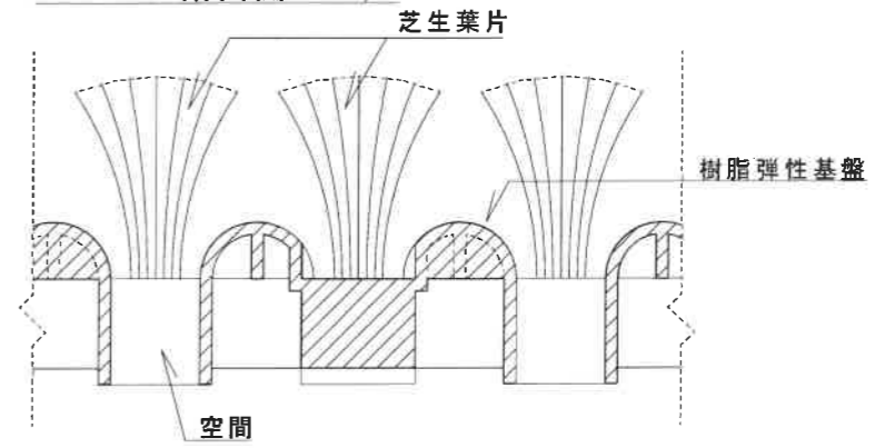
B-B' 断面図 S=1/1
