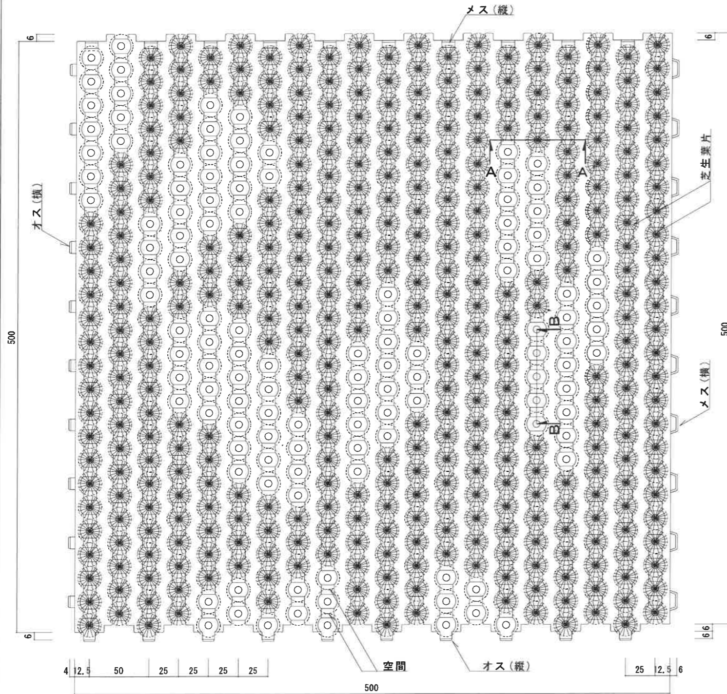
平面図 S=1/3
