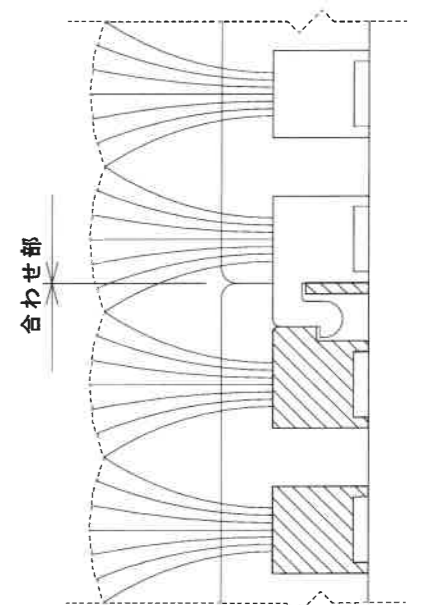
縦方向連結 S=1/1
