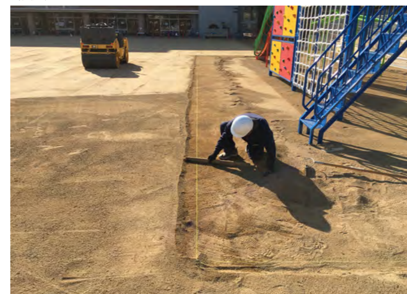
鋤取り整地
