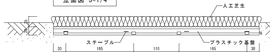
立面図 S=1/4
