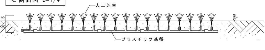
右側面図 S=1/4
