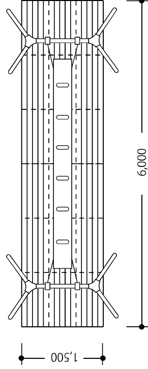
遊動円木 (9㎡)
