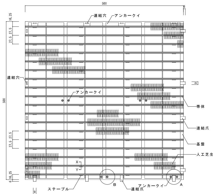
立面図 S=1/4
