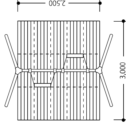
2連ブランコ (7.5㎡)
