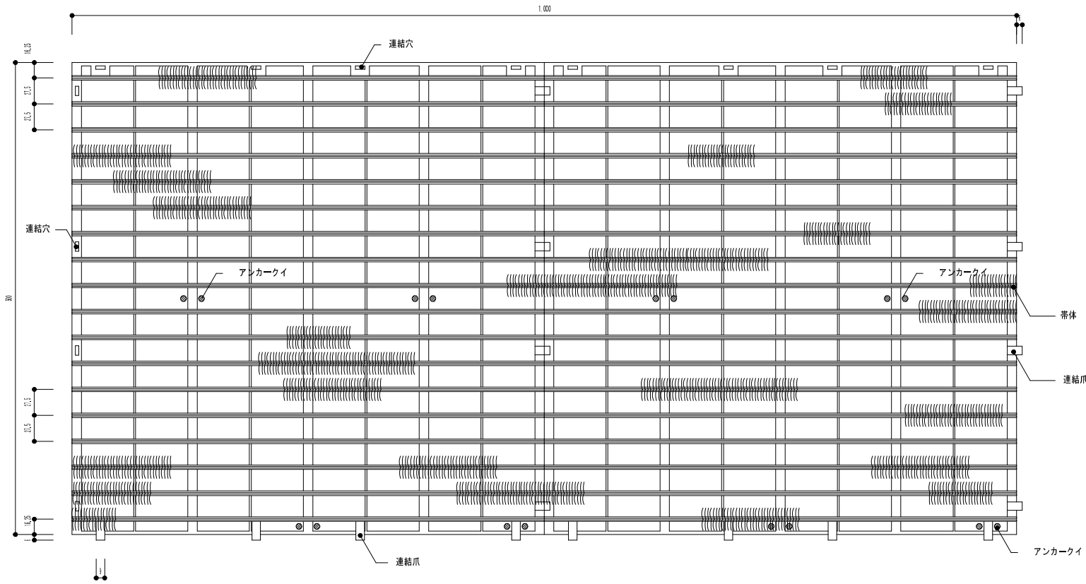
立面図 S=1/4
